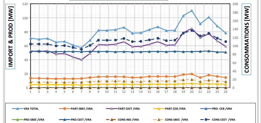
COURBES DE CHARGE ILOT VRA
