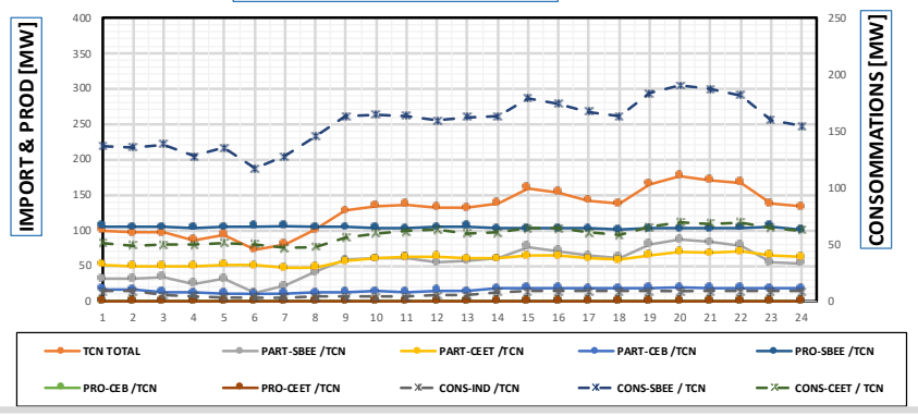
COURBES DE CHARGE ILOT TCN
